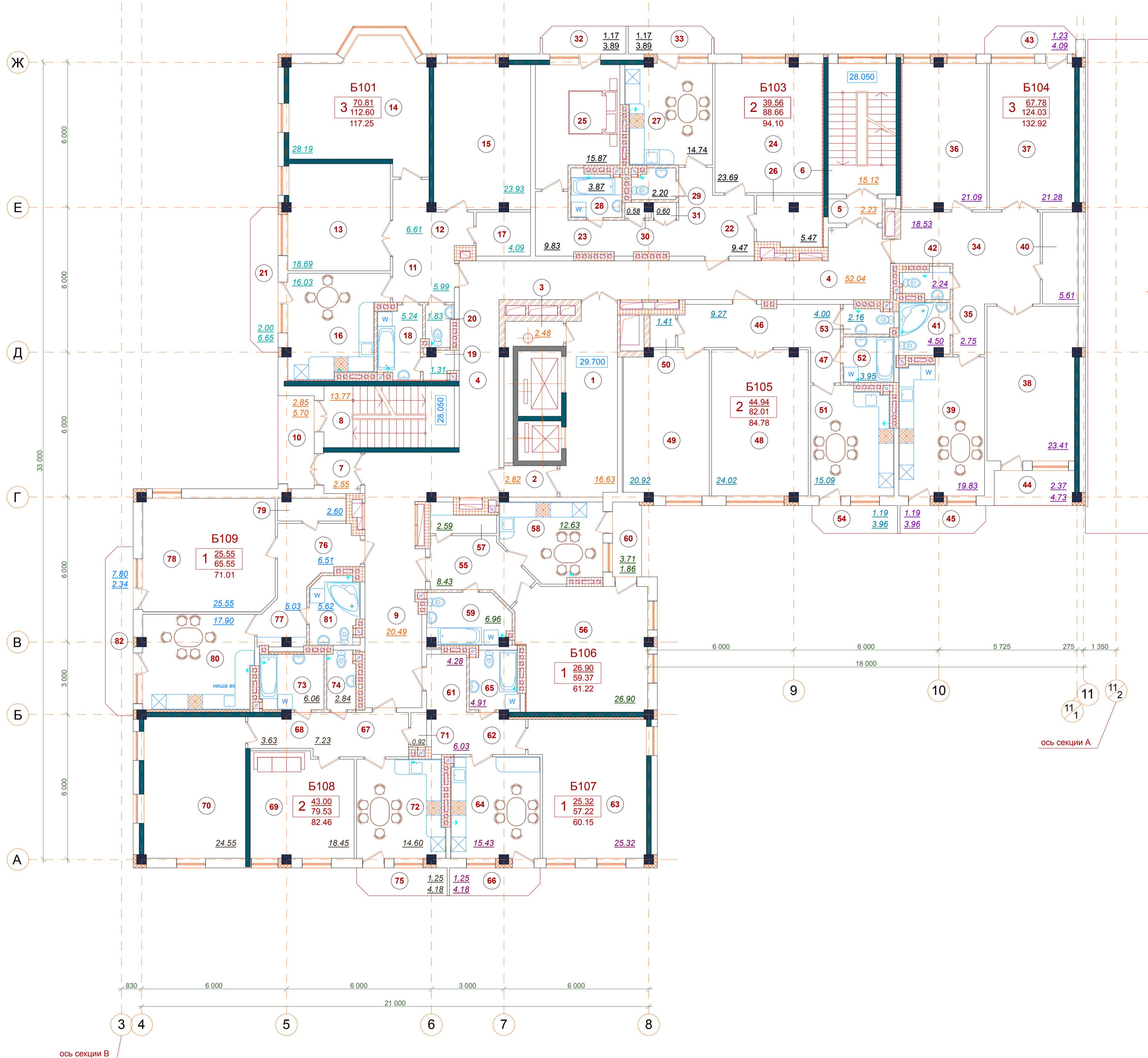
ПЛАН НА ОТМ. 29.700; (10-ЫЙ ЭТАЖ)
